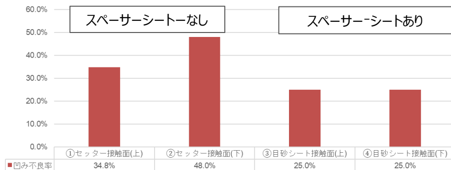
【セッター接触基板凹み不良比較】
