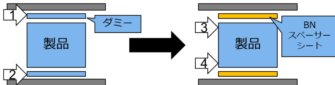
【セッター接触基板凹み不良比較】
